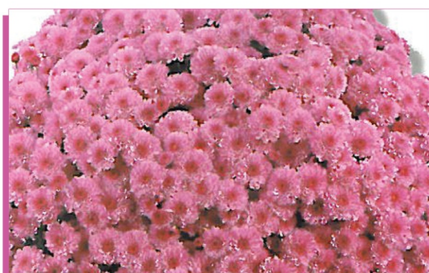
Boreliae
